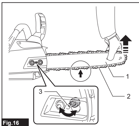
Fig.16 ► 1. Barra de guía 2. Cadena de la sierra 3. Tornillo de ajuste de la cadena
